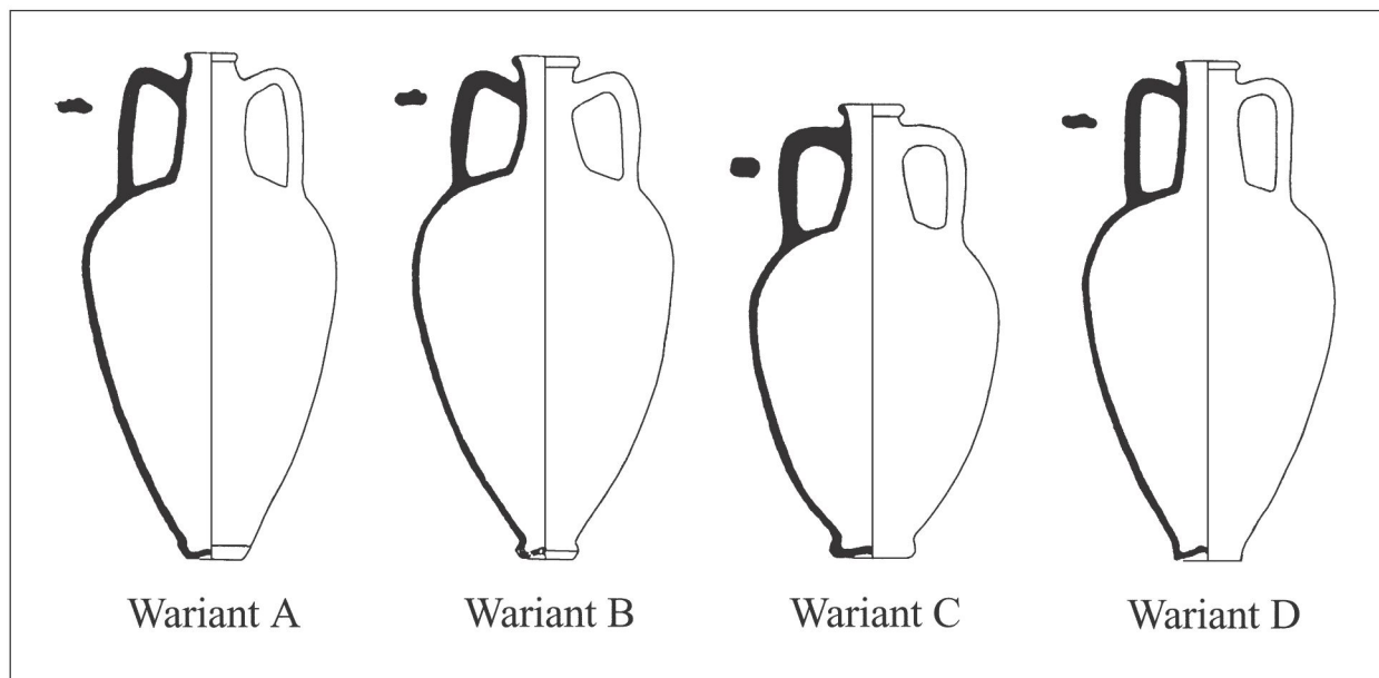
Fig. 4. Warianty amfor Forlimpopoli wydzielone przez T. Aldini'ego, wg ALDINI 1978: fig. 2
