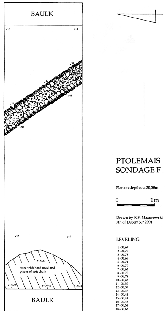
Fig. 48. Plan sondażu F (rys. R.F. Mazurowski)
