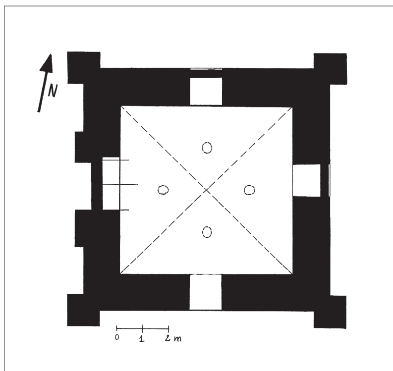
Fig. 3. Plan „Piramidy Żabińskiej” (na podstawie rysunku D. M. Ambrosiewicza).
