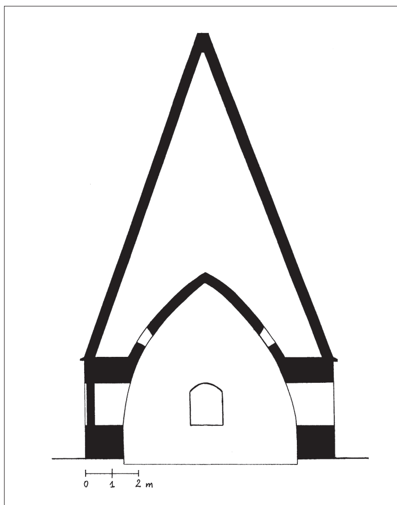
Fig. 4. Przekrój „Piramidy Żabińskiej” (na podstawie rysunku D. M. Ambrosiewicza).
